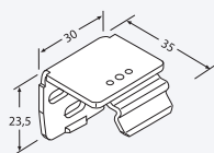
Настенный кронштейн 58201 белый
