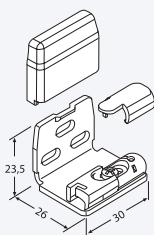
Настенный кронштейн с держателем нити 58231 белый
