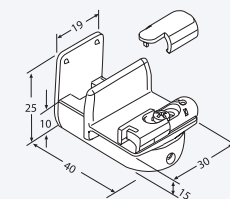
Клеммный кронштейн с держателем нити 58331 белый
