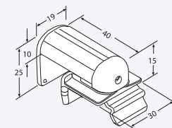
Клеммный кронштейн 58301 белый
