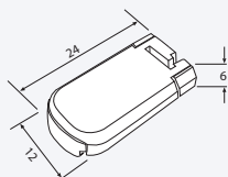
Держатель нити 58131 белый
